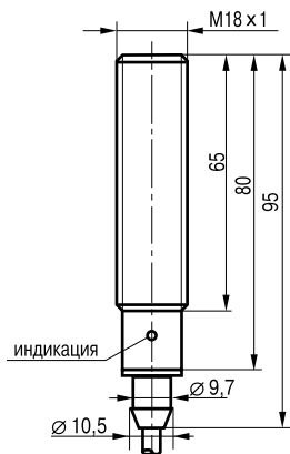
Габаритный чертеж.
